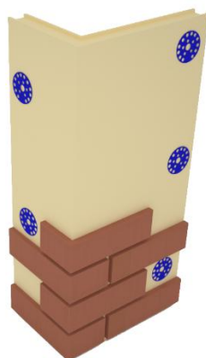
FIGUUR 2C: VERSCHILLENDE TYPES HOEKEN MET HOEKBAKSTEENSTRIPS (BEKLEDING MET BAK- OF KERAMISCHE STEENSTRIPS)
