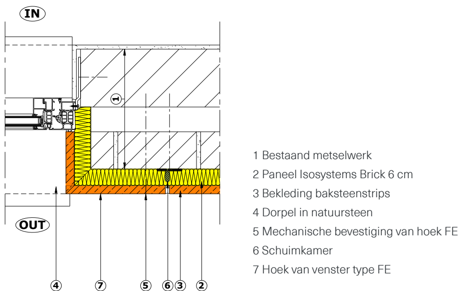
Afwerkingsdetails van de vensteropeningen met blauwe steen
